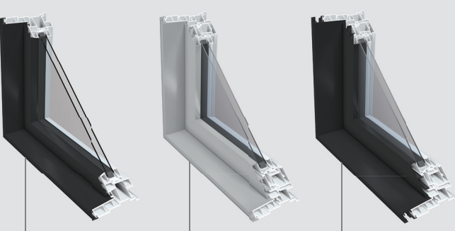
Cadre 5 3/4" Fixe plat Noir Cadre 5 3/4" Volet plat Anodisé clair Cadre 6 9/16" Volet plat Noir
