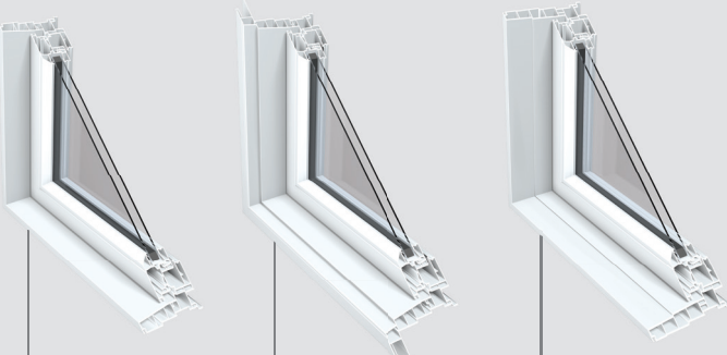
Cadre 5 1/4" Volet plat Sans moulure Cadre 6 1/4" Volet plat Moulure intégrée Cadre 6 9/16" Volet plat Sans moulure
